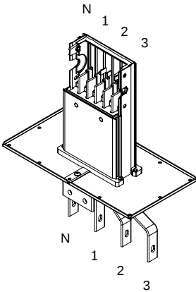
Тип 1 без соединительного элемента
